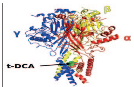
Homologie-Modell von humanem \alpha\beta\gamma ENaC mit angelagerter Taurodeoxycholsäure (t-DCA) in einer durch Computersimulation (molekular docking) vorhergesagten Position in der Porenregion des Kanals
