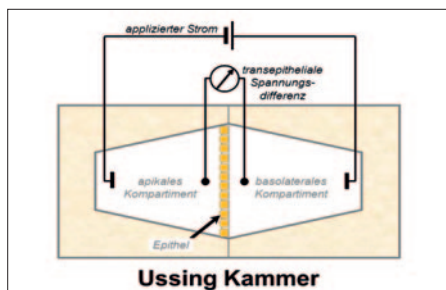
Schematische Darstellung einer sogenannten Ussing-Kammer für Kurzschlussstrommessungen zur Quantifizierung des elektrogenen transepithelialen Ionentransports
