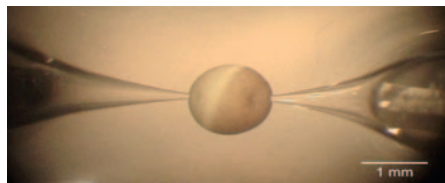
Xenopus laevis Oozyte mit zwei eingestochenen Mikroelektroden zur Messung von Ganzzellströmen mit Hilfe der TEVC-Technik
